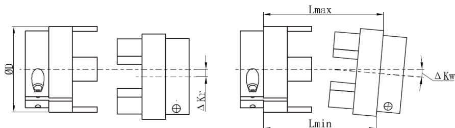
Схема возможных несоосностей муфты с упругим элементом «звездочка»
