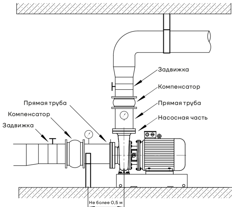
Рис. 12 Схема подключения насоса
