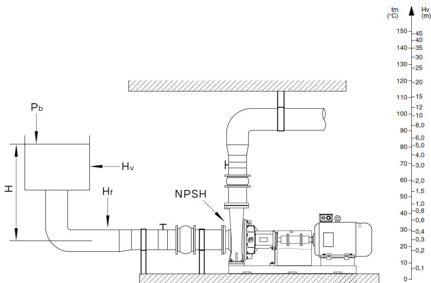
Рис. 7 Система с насосом
