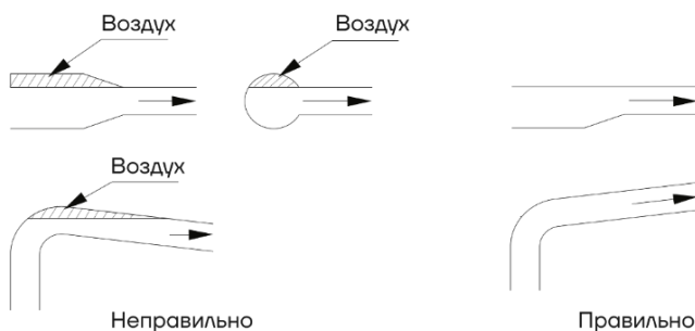
Рис. 11 Правильный монтаж трубопроводов
